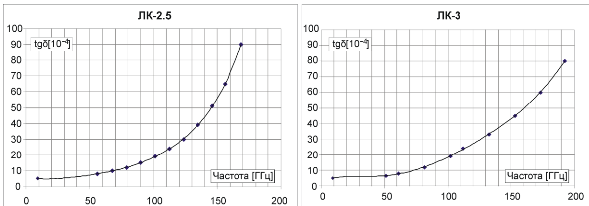
Рис. 3. Зависимость \text{tg}\delta от частоты пенно-керамик ЛК-2.5 и ЛК-3. Аппроксимация – полиномы 6-й степени. В пределах ошибки измерения не выявлена анизотропия показателя преломления. Для ЛК-2.5: показатель преломления возрастает практически линейно от n (9.4 ГГц) = 1.58 до n (170 ГГц) = 1.61. Для ЛК-3: величина показателя преломления меняется практически линейно от n (9.4 ГГц) = 1.73 до n (192 ГГц) = 1.77.
