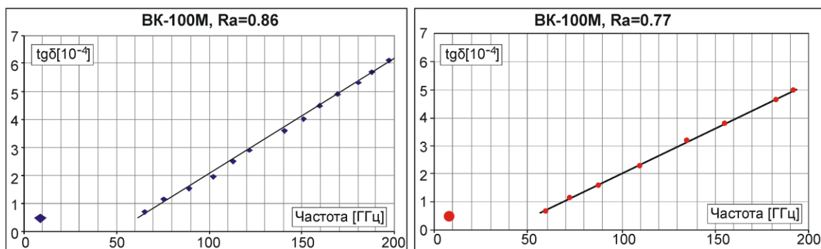
Рис. 5. Зависимость \text{tg}\delta от частоты двух образцов керамики BK-100M с разной шероховатостью Ra (мкм). Зависимость близка к линейной в ММ диапазоне, но не совпадает с измерениями на СВЧ. Несовпадения указывает, что на низких частотах другой механизм поглощения. Это подтверждается различием в величине показателя преломления. На 9.4 ГГц n = 3.194 , в ММ диапазоне, в пределах ошибки измерений, n=3.165 . Для обоих образцов выявлена небольшая анизотропия показателя преломления: отличие двух взаимно перпендикулярных поляризаций в пределах 0.001.
