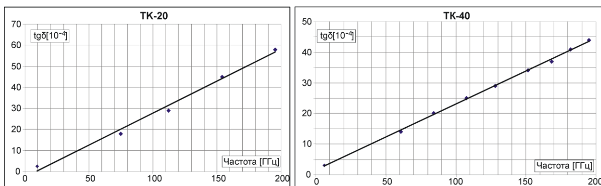
Рис. 2. Зависимость \text{tg}\delta от частоты керамических материалов ТК-20 и ТК-40. Зависимость близка к линейной, включая результаты измерений на СВЧ. В пределах ошибки измерения не выявлена анизотропия показателя преломления. Для ТК-20: показатель преломления возрастает практически линейно от n(9.4 \text{ ГГц}) = 4.404 до n(200 \text{ ГГц}) = 4.416 . Для ТК-40: n(60-200 \text{ ГГц}) = 6.255 \pm 0.001 , n(6 \text{ ГГц}) = 6.316 .
