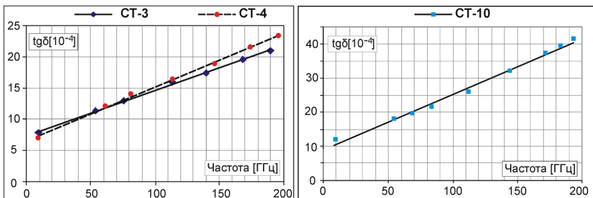
Рис. 4. Зависимость \text{tg}\delta от частоты керамических материалов СТ-3, СТ-4 и СТ-10.
