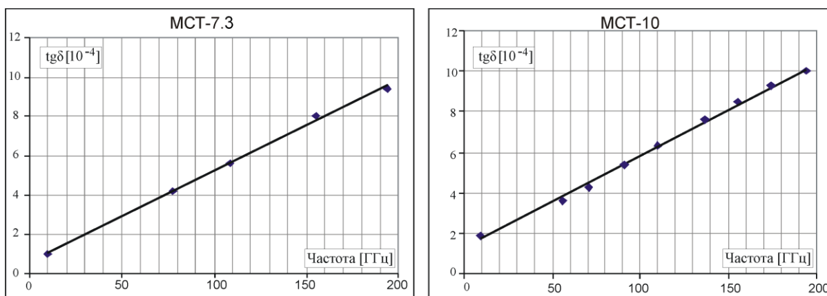
Рис. 1. Зависимость \text{tg}\delta от частоты керамических материалов МСТ-7.3 и МСТ-10. Зависимость близка к линейной, включая результаты измерений на СВЧ. В пределах ошибки измерения не выявлена анизотропия показателя преломления. Для МСТ-7.25: n(80-200 \text{ ГГц}) = 2.658 \pm 0.001 , n(9.4 \text{ ГГц}) = 2.72 . Для МСТ-10: n(55-200 \text{ ГГц}) = 3.1855 \pm 0.001 , n(9.4 \text{ ГГц}) = 3.225 .
