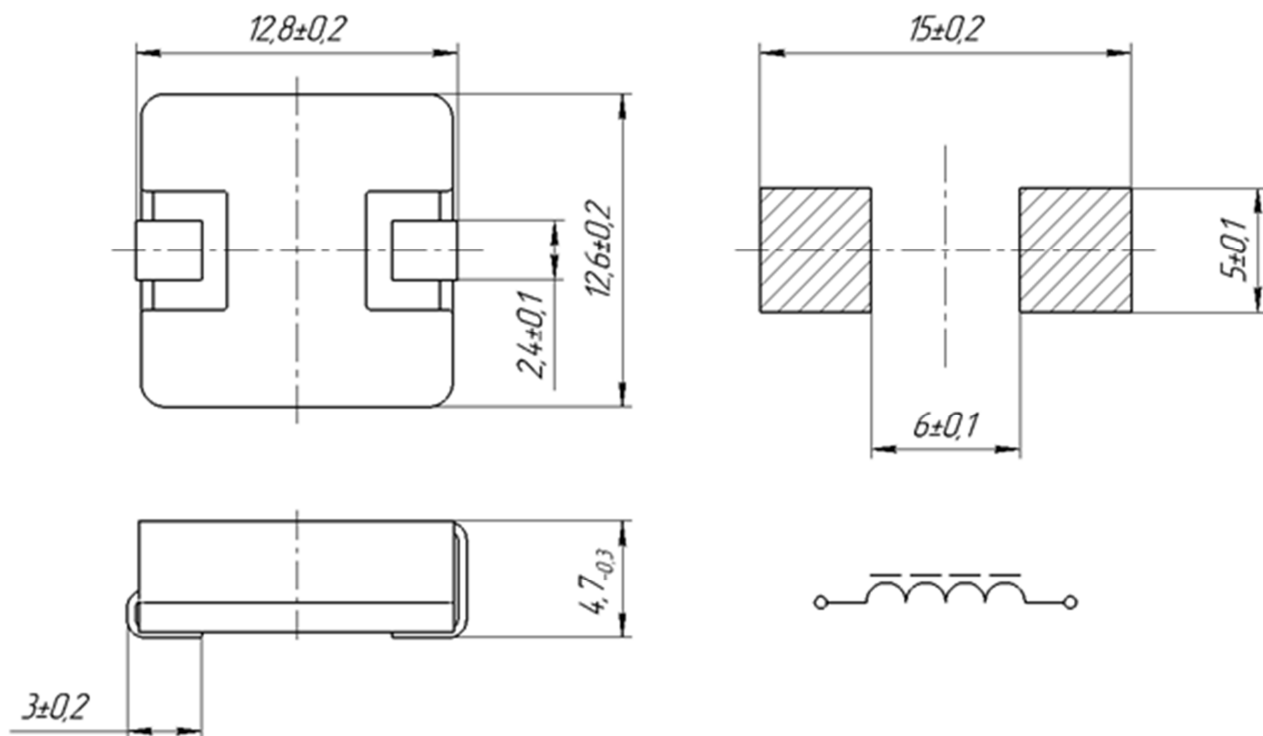
Дроссель Д372-20
