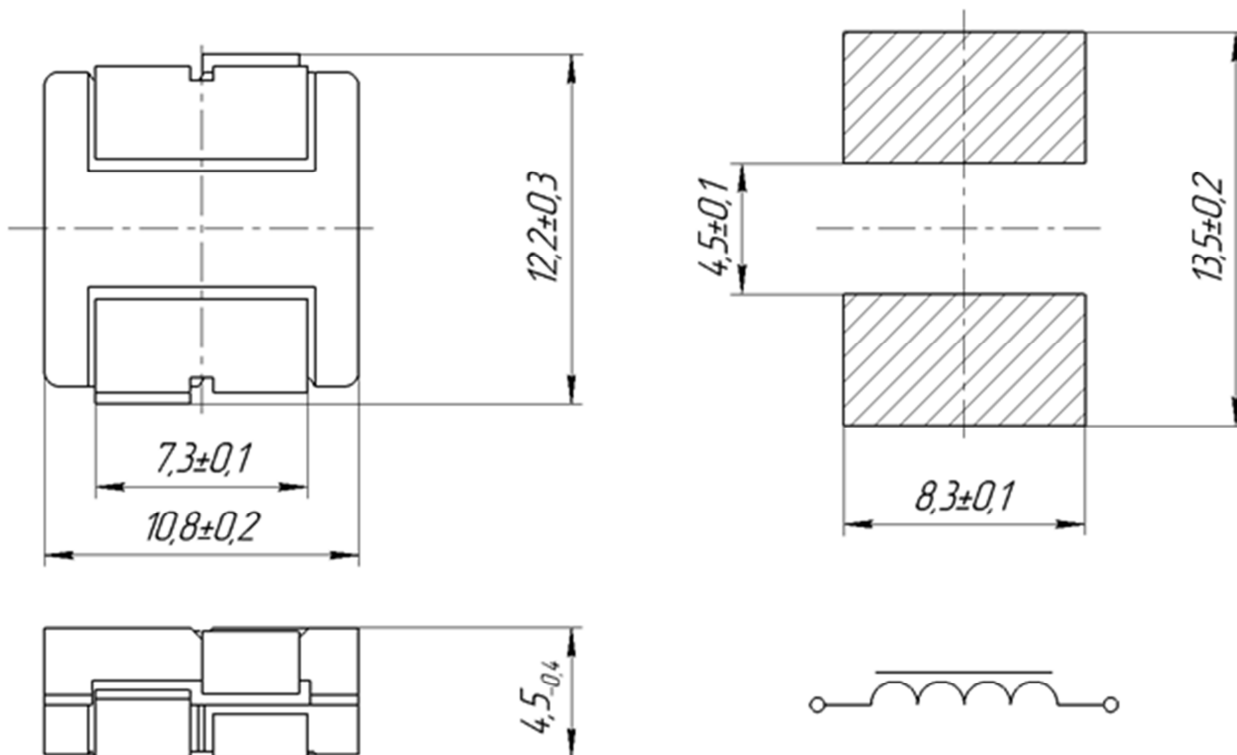
Дроссель Д372-19
